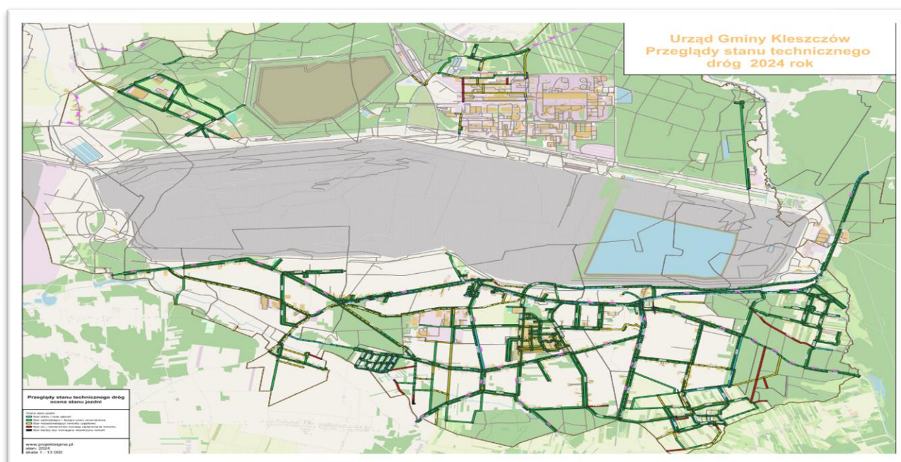
Rysunek 3. Mapa stanu technicznego dróg gminnych na podstawie przeglądu podstawowego i rozszerzonego 2024
